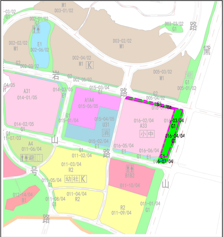
修改前土地利用规划图
